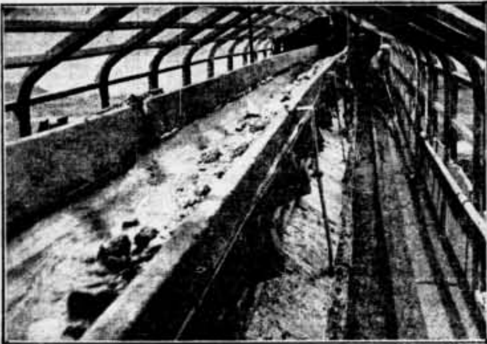
Vista general de la instal·lació i anoves de la draga de l'exploració de Missa, a l'Ural
